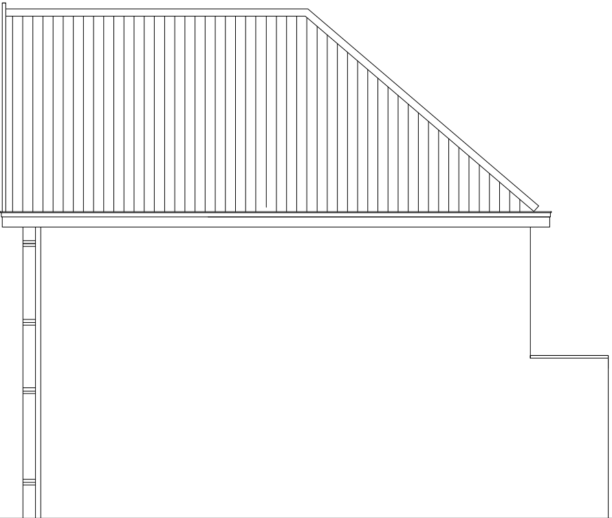
Zijgevel Woning 2 & 4
